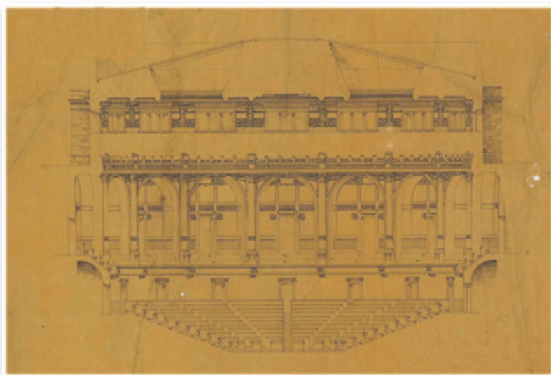
Ampliamento del Palazzo di Montecitorio. Sezione trasversale dell'Aula. Tav. XIX, 28 novembre 1905.
