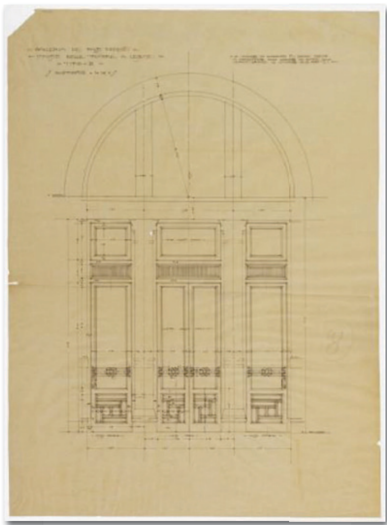
"Galleria dei passi perduti. Imposte delle trifore a lesene tipo B" [1909 - 1923]. ASCD, Fondo Ernesto Basile
